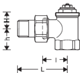
Rys. 5 Wykonanie kątowe – E
