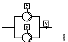
Sterowanie pompą bliźniaczą z nadzorem przepływu i przeciążenia
