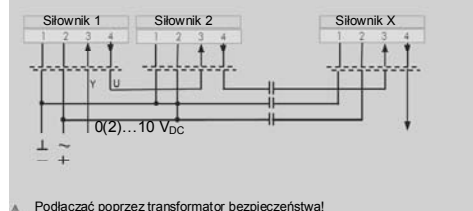
Schemat połączeń przy pracy równoległej FSAM24.2
