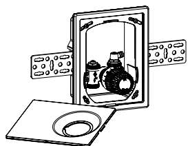
Multibox Eclipse RTL z ogranicznikiem temperatury powrotu (RTL)
